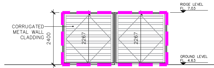
5 Existing Container Structure F1 - Section A-A EX-F-100 1:100
