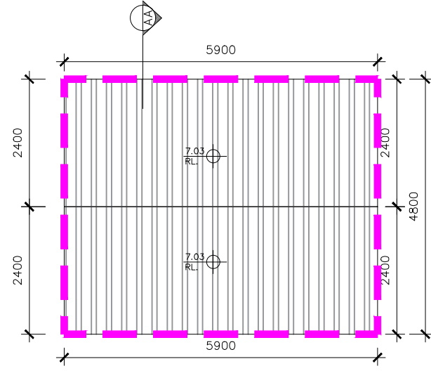
2 Existing Container Structure F1 - Roof Plan EX-F-100 1:100
