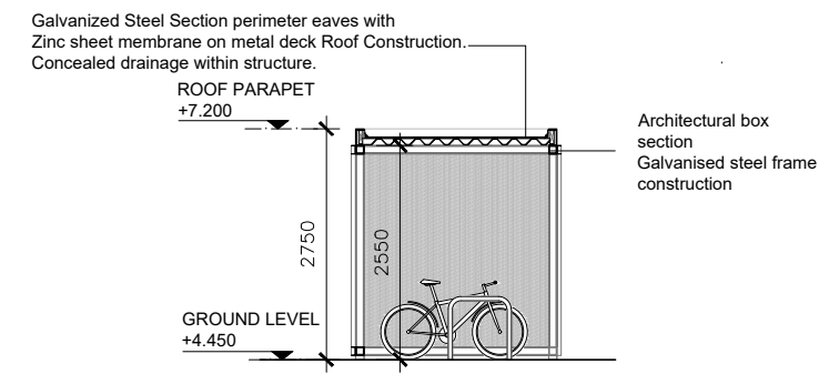
06 Section A-A PA-402 1:100
